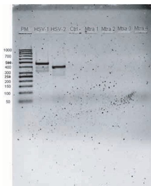
Figura 2. Productos de PCR para detección de HSV-1 y HSV-2. PM = marcador de peso molecular, HSV-1 = control positivo para HSV-1, HSV-2 = control positivo para HSV-2, Ctr1- control negativo, Mtra 1, 2, 3 y 4 = muestras negativas a HSV-1 y HSV-2.
